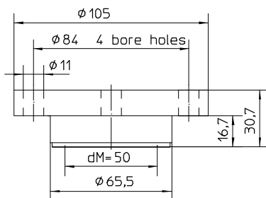
DRD-connection DN50 PN40 *
